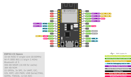
图 8: ESP32-C3-DevKitC-02 管脚布局 (点击放大)
