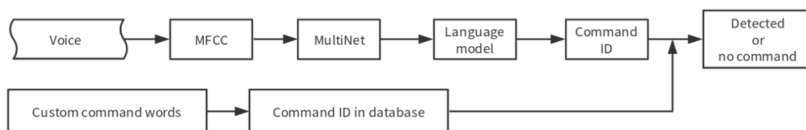
图 1: speech_command-recognition-system
