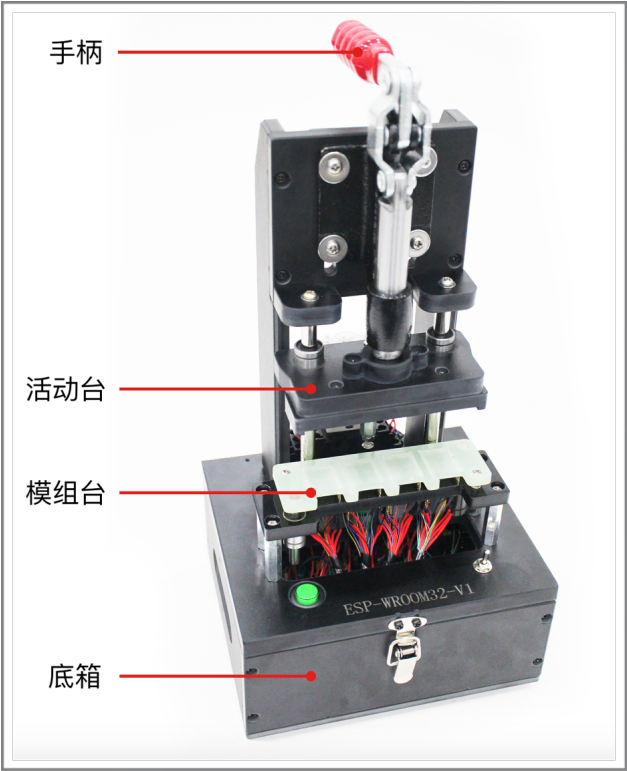
图 89: 模组治具机构示意图 (ESP-WROVER)
