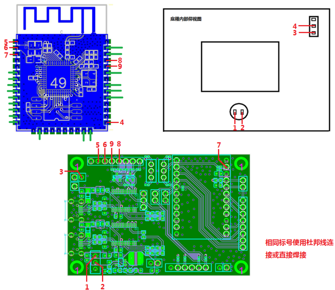
图 98: ESP-WROVER 模组台接线示意图
