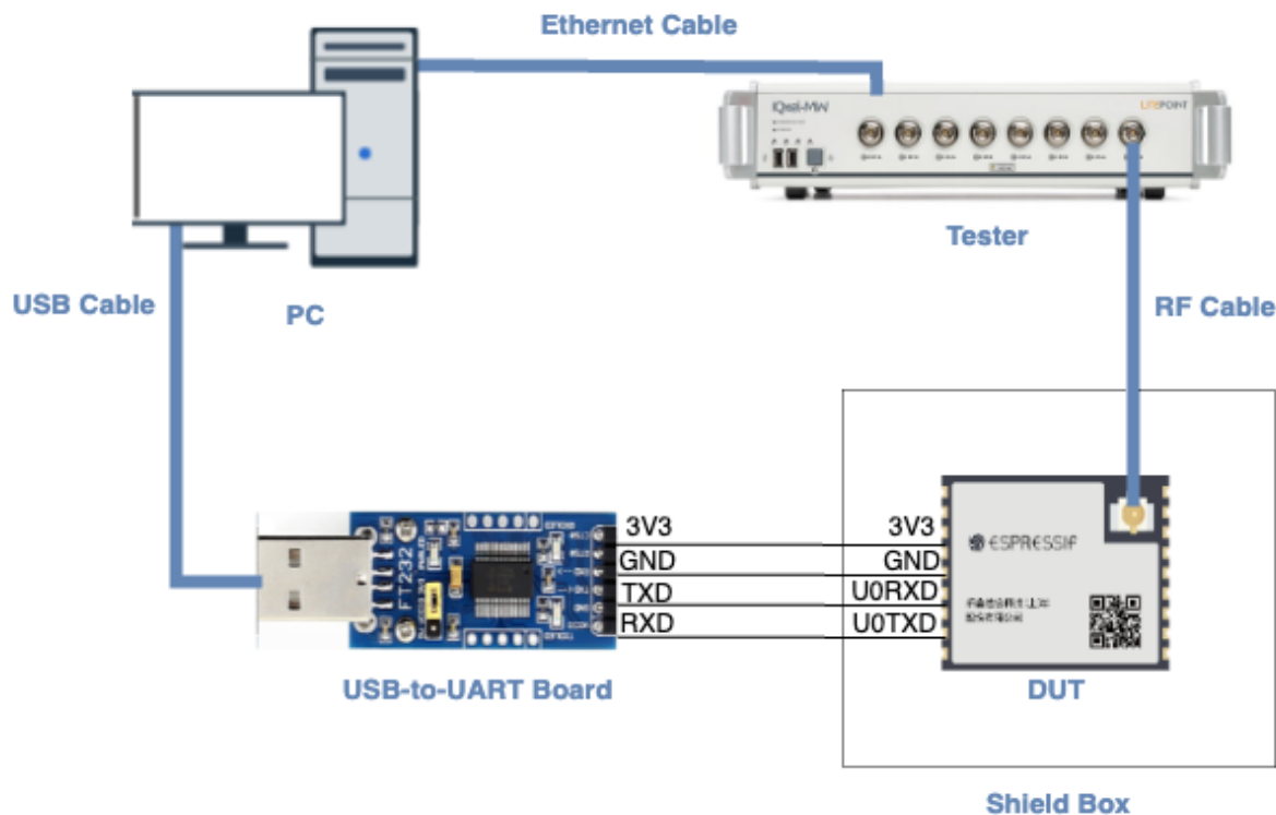
图 44: 测试环境搭建示意图
