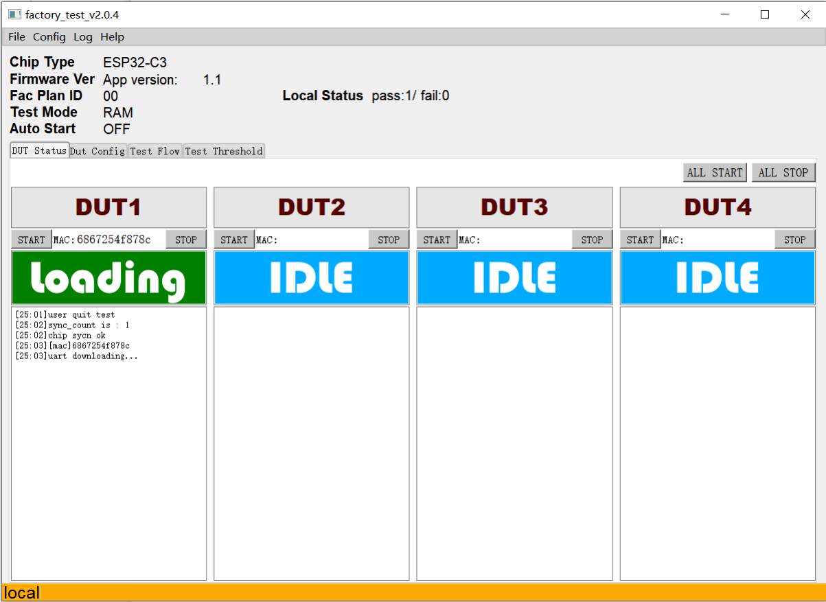
图 84: 同步过程
