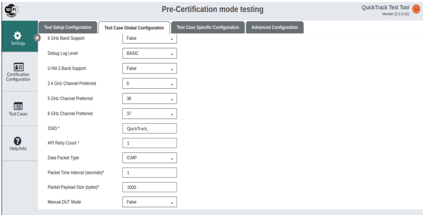
图 62: QuickTrack 设置-2
