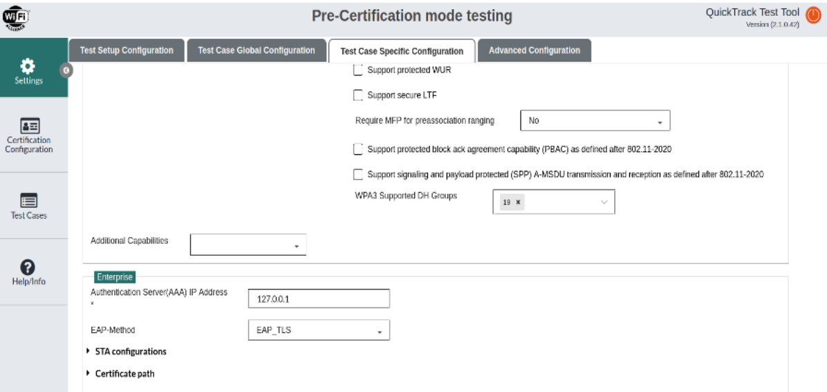
图 64: QuickTrack 设置-4
