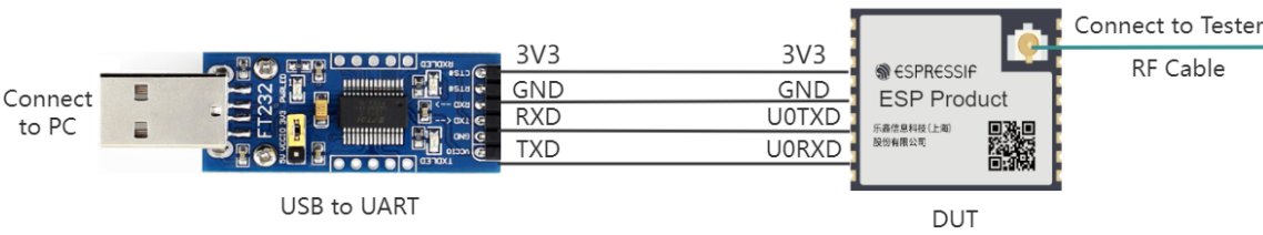
图 19: UART 连接说明
