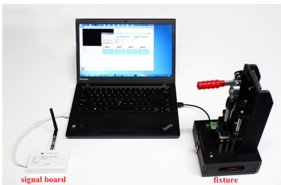
图 75: 信号板方案的实物连接
