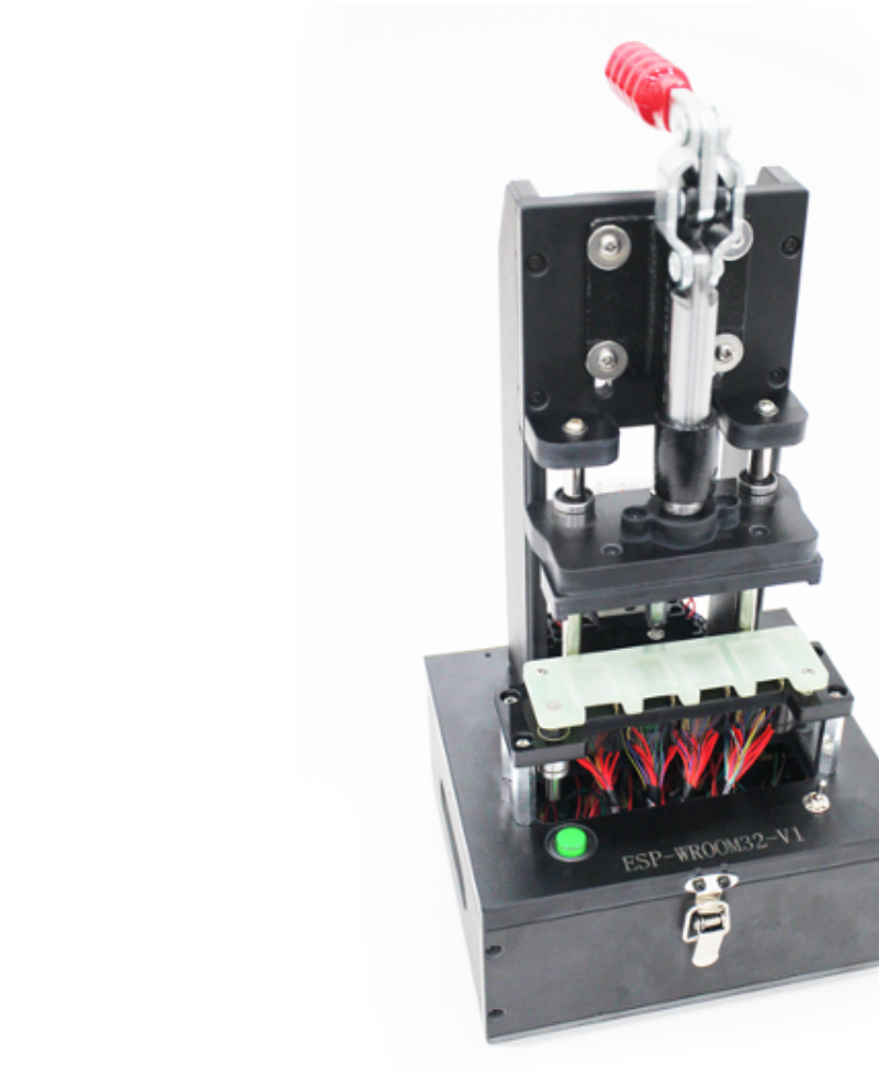
图 77: 治具整体外观
