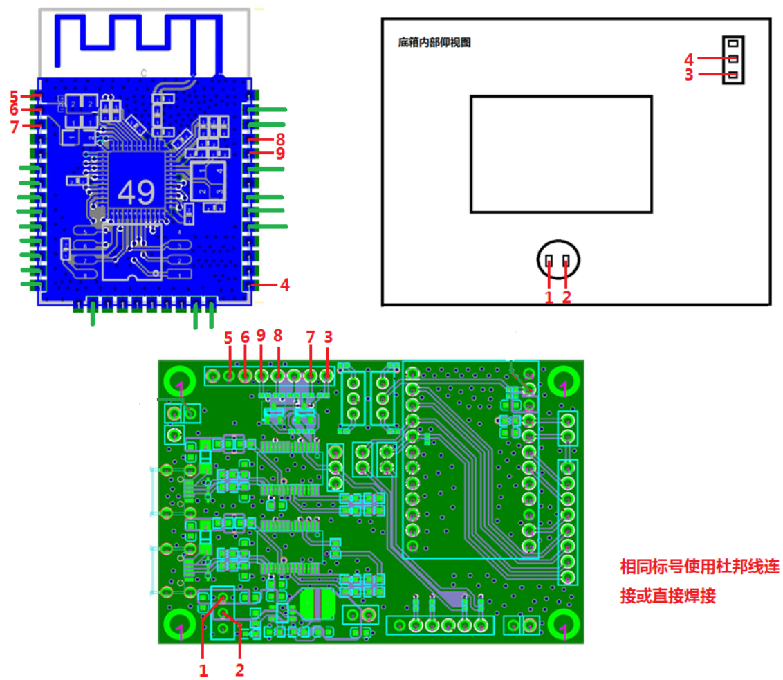
图 100: ESP-WROOM-32 模组台接线示意图
