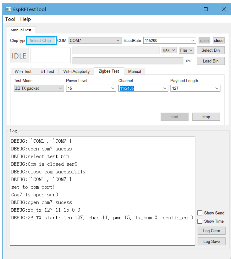
图 47: Zigbee 发射性能测试
