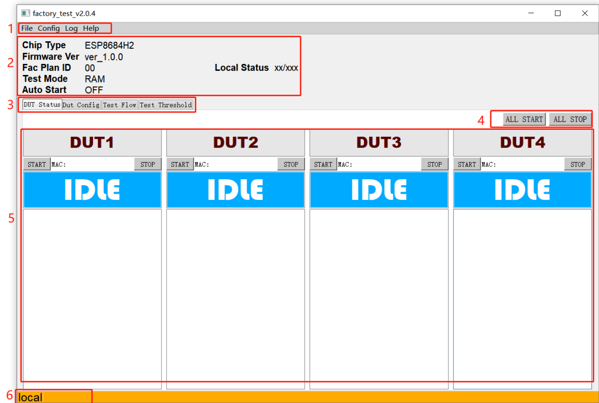
图 78: 工具主界面
