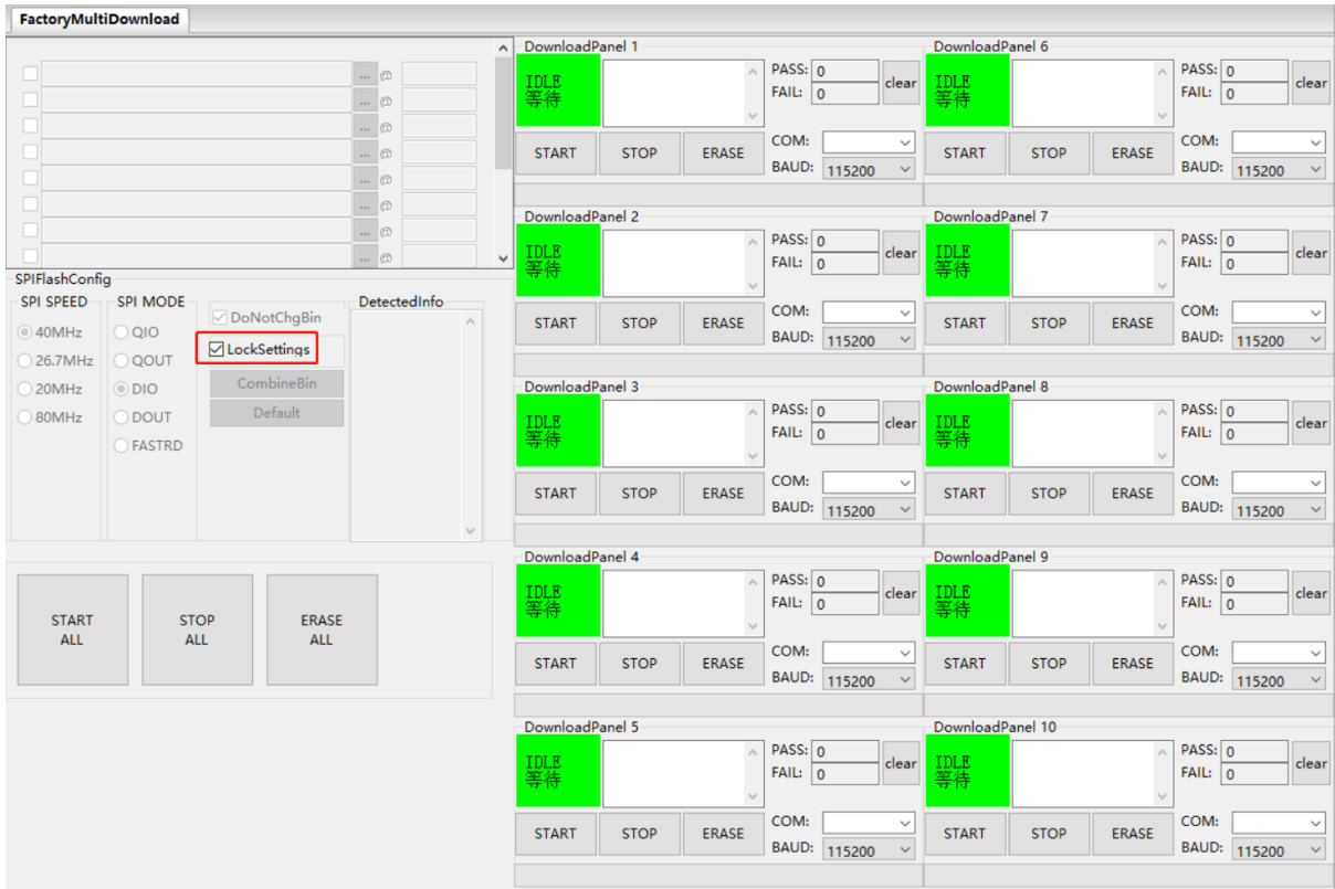
图 68: FactoryMultiDownload 界面
