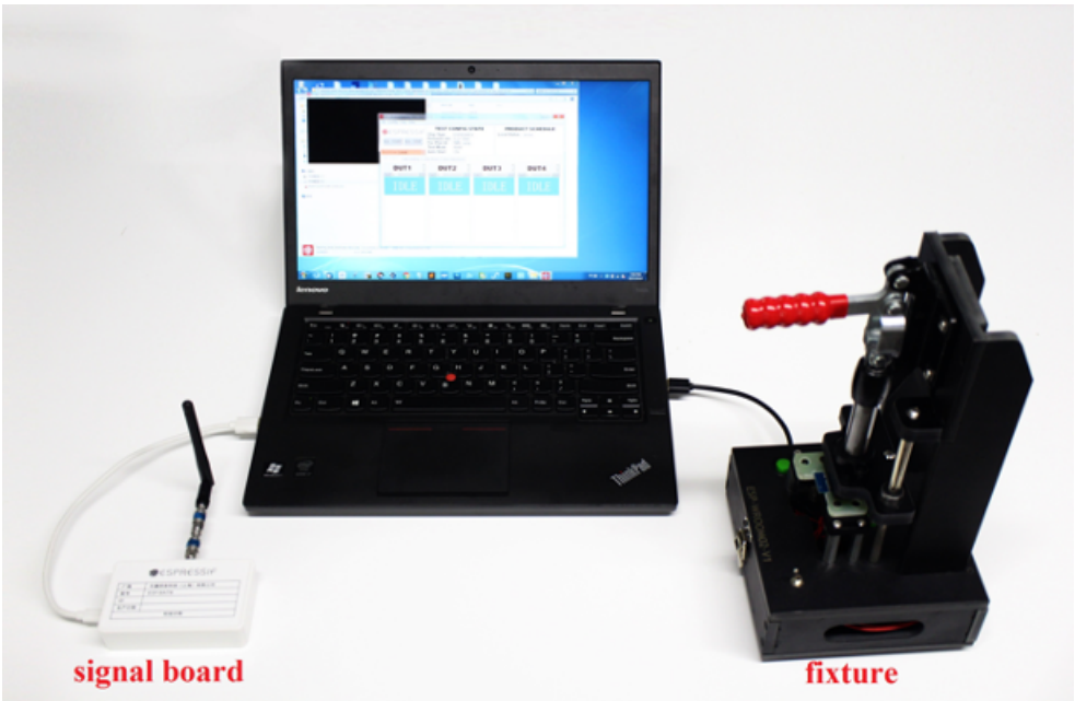
图 75: 信号板方案的实物连接
