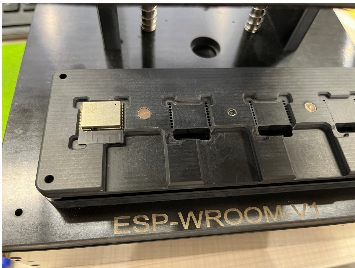
图 93: ESP-WROOM 治具模组台
