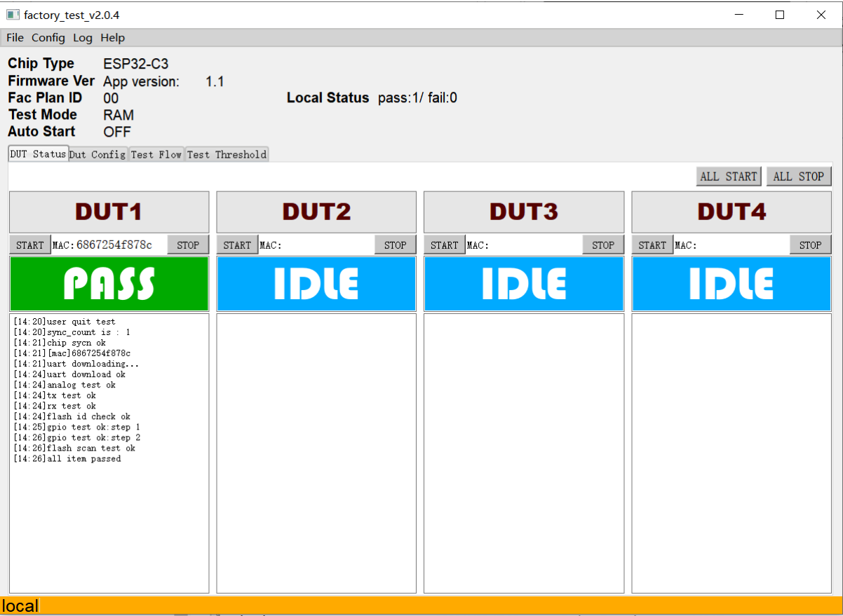
图 88: 测试完成
