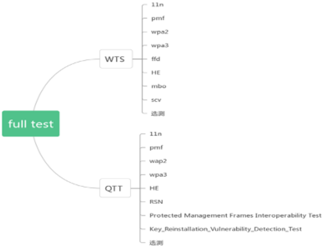
图 51: full-test 测试项
