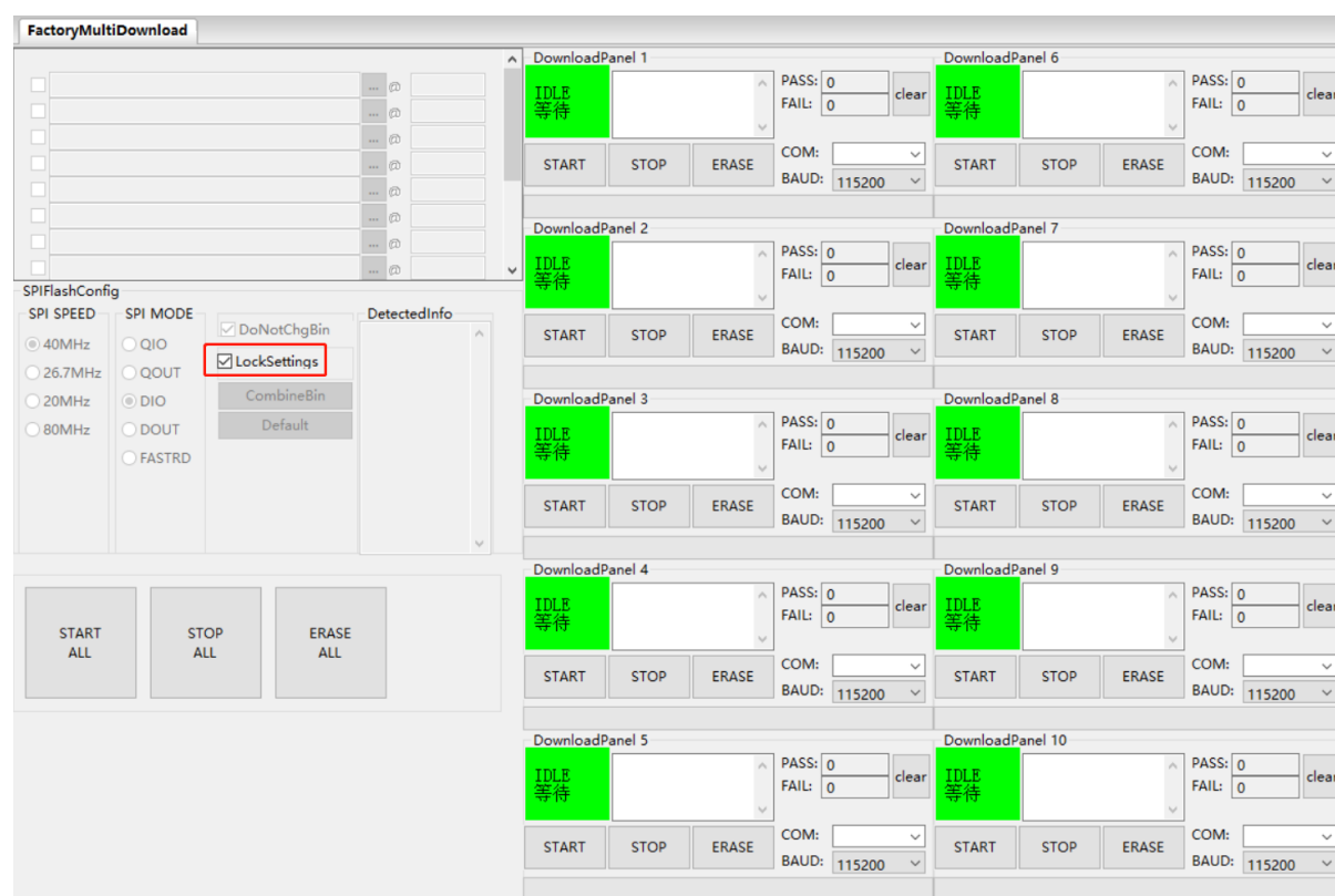
图 68: FactoryMultiDownload 界面
