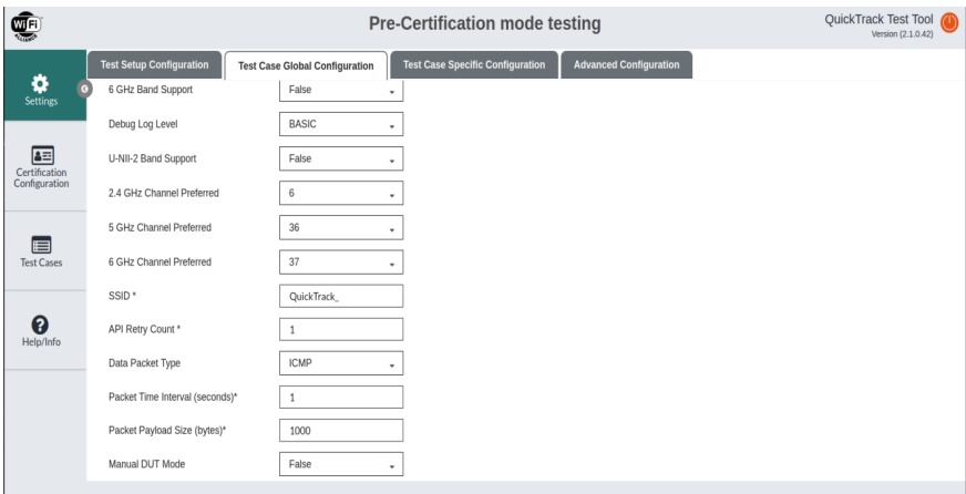
图 62: QuickTrack 设置-2
