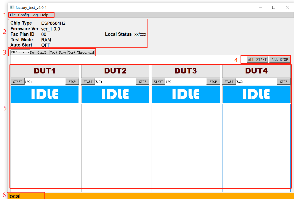
图 80: 工具主界面
