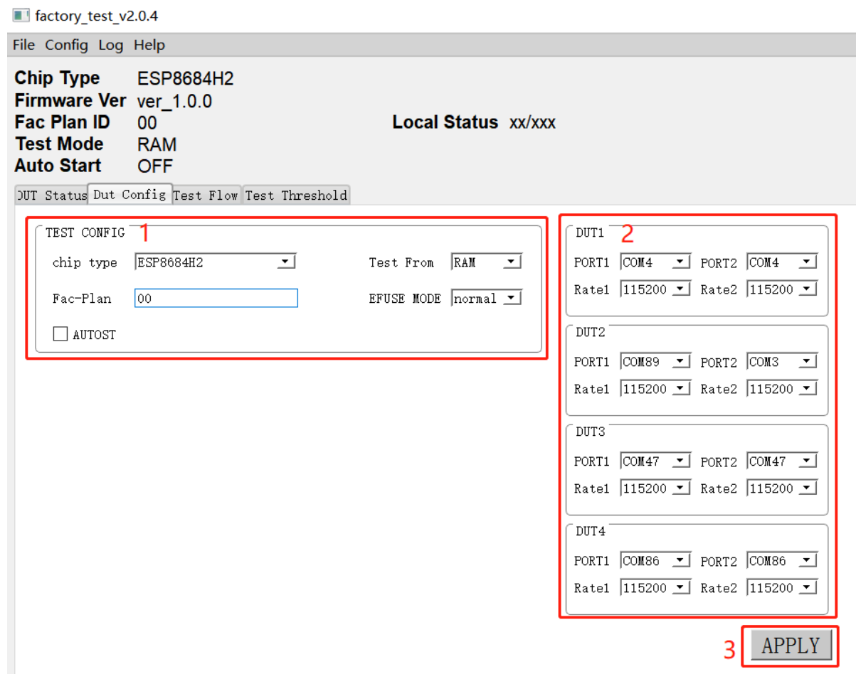
图 74: DUT Config 配置界面
