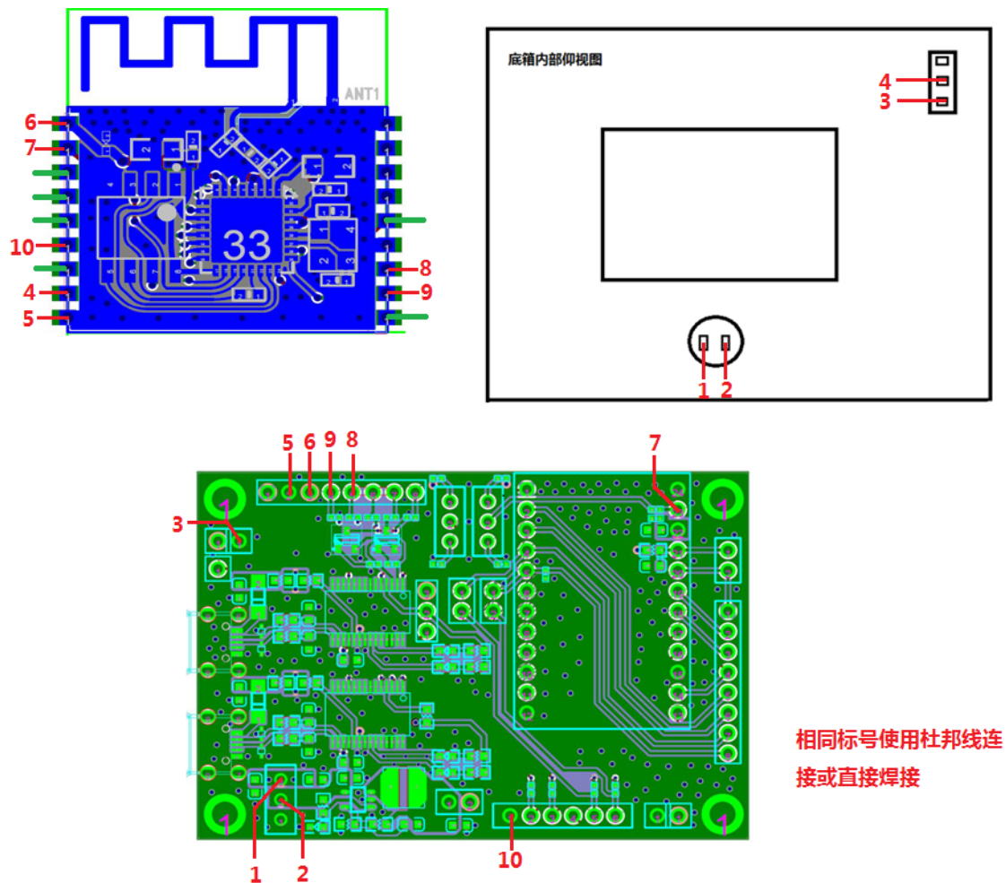
图 91: ESP-WROOM-02 模组台接线示意图
