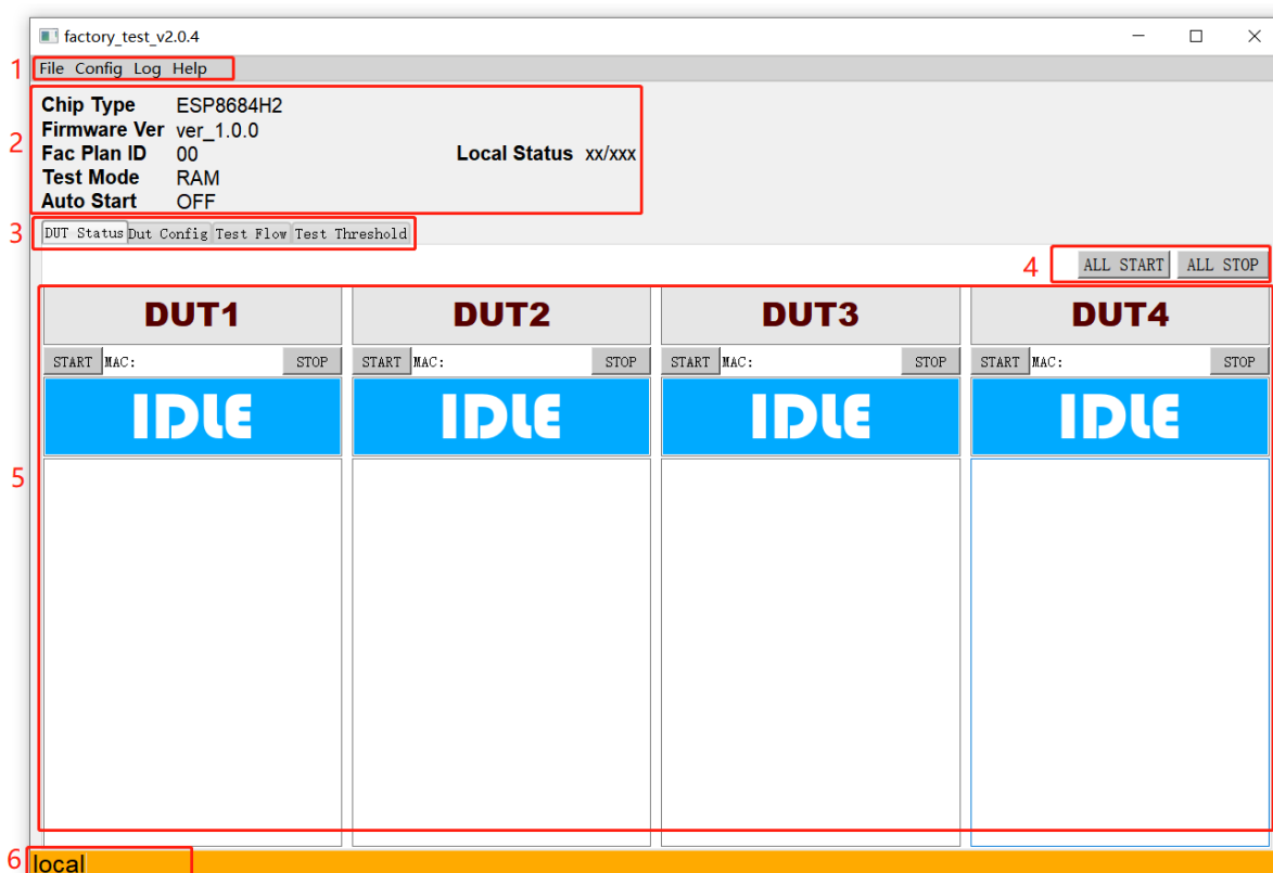
图 73: 工具主界面
