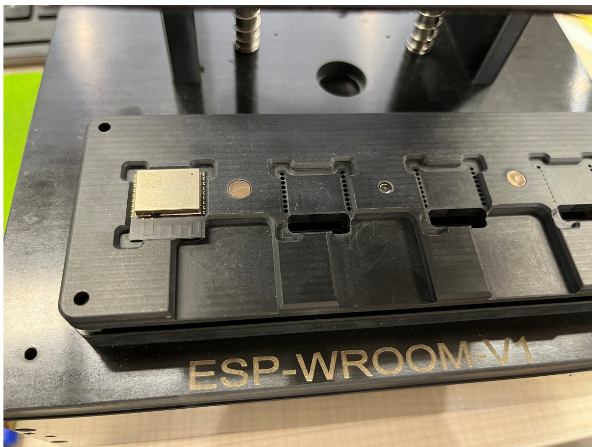
图 85: ESP-WROOM 治具模组台
