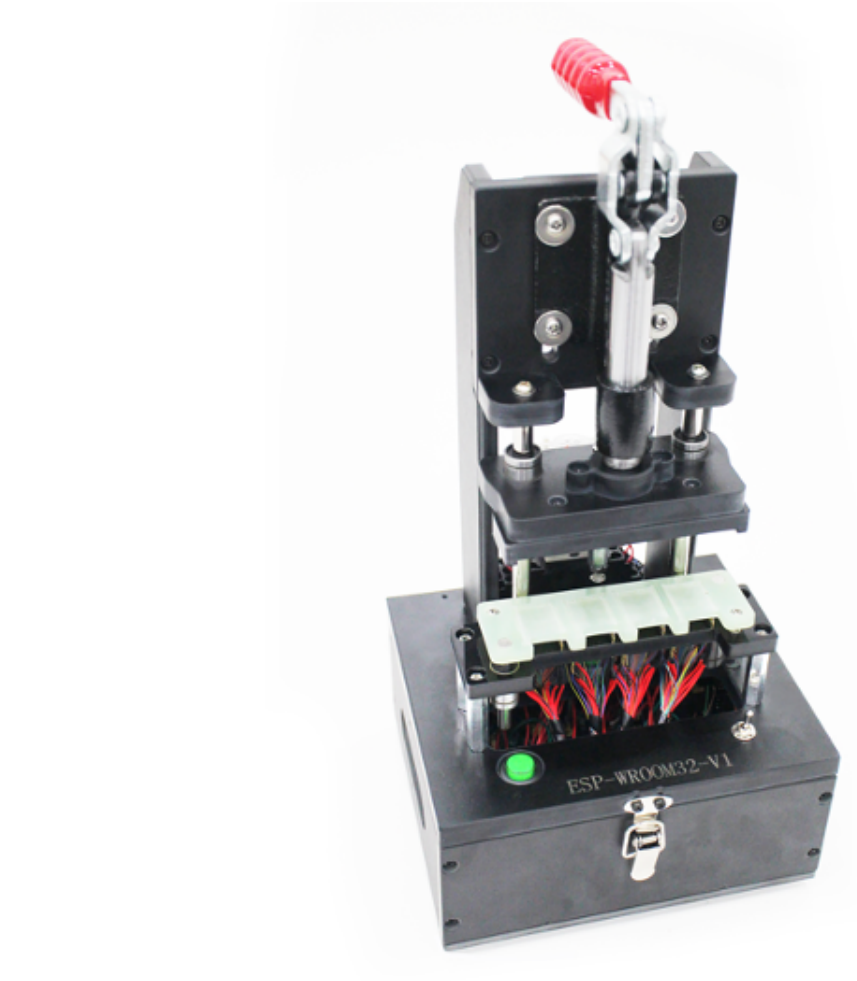
图 72: 治具整体外观
