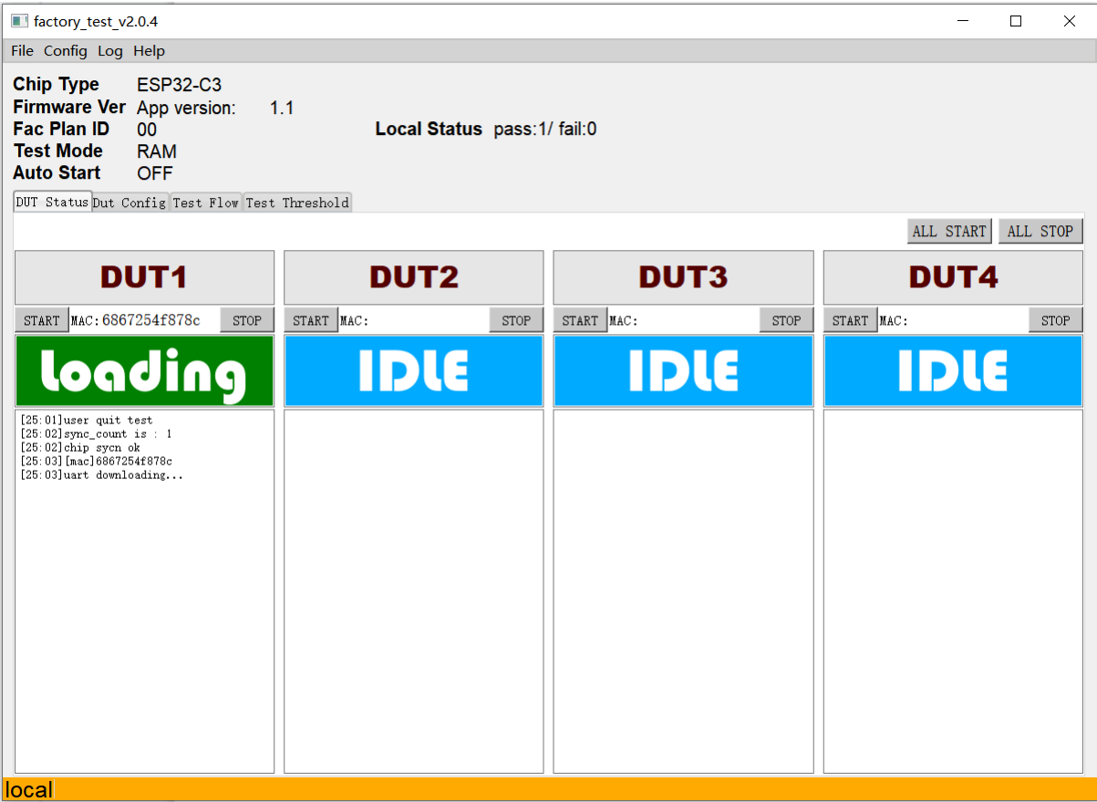
图 79: 同步过程
