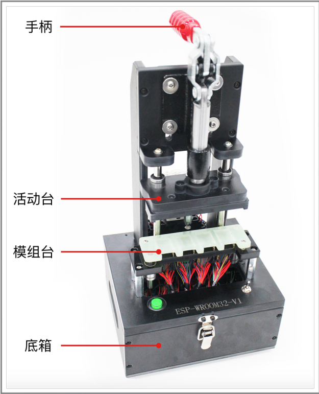
图 84: 模组治具机构示意图 (ESP-WROVER)
