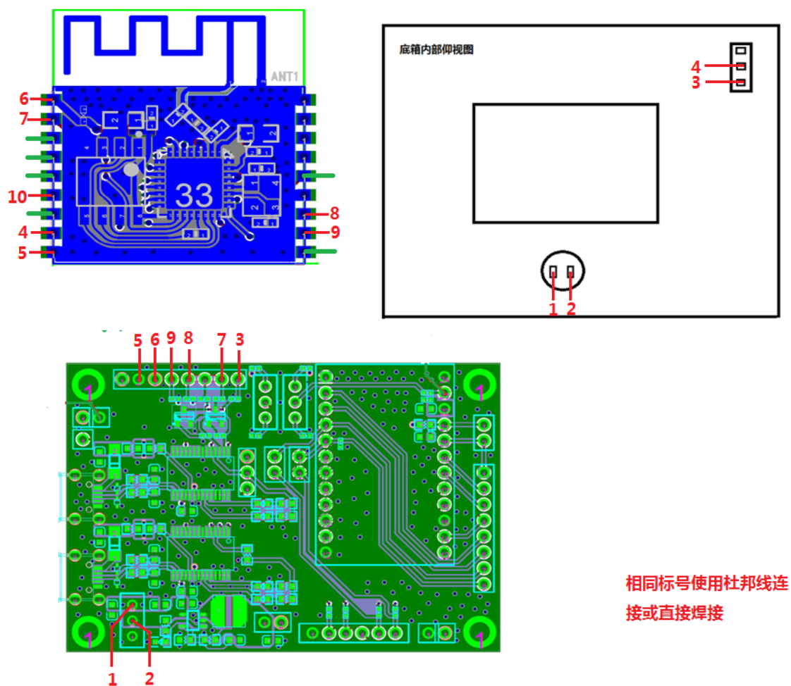
图 70: ESP-WROOM-02 模组台接线示意图
