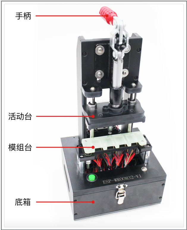
图 60: 模组治具机构示意图 (ESP-WROVER)
