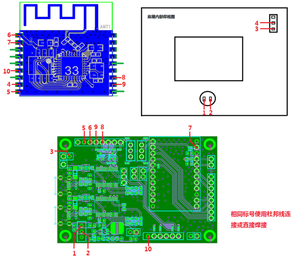
图 67: ESP-WROOM-02 模组台接线示意图
