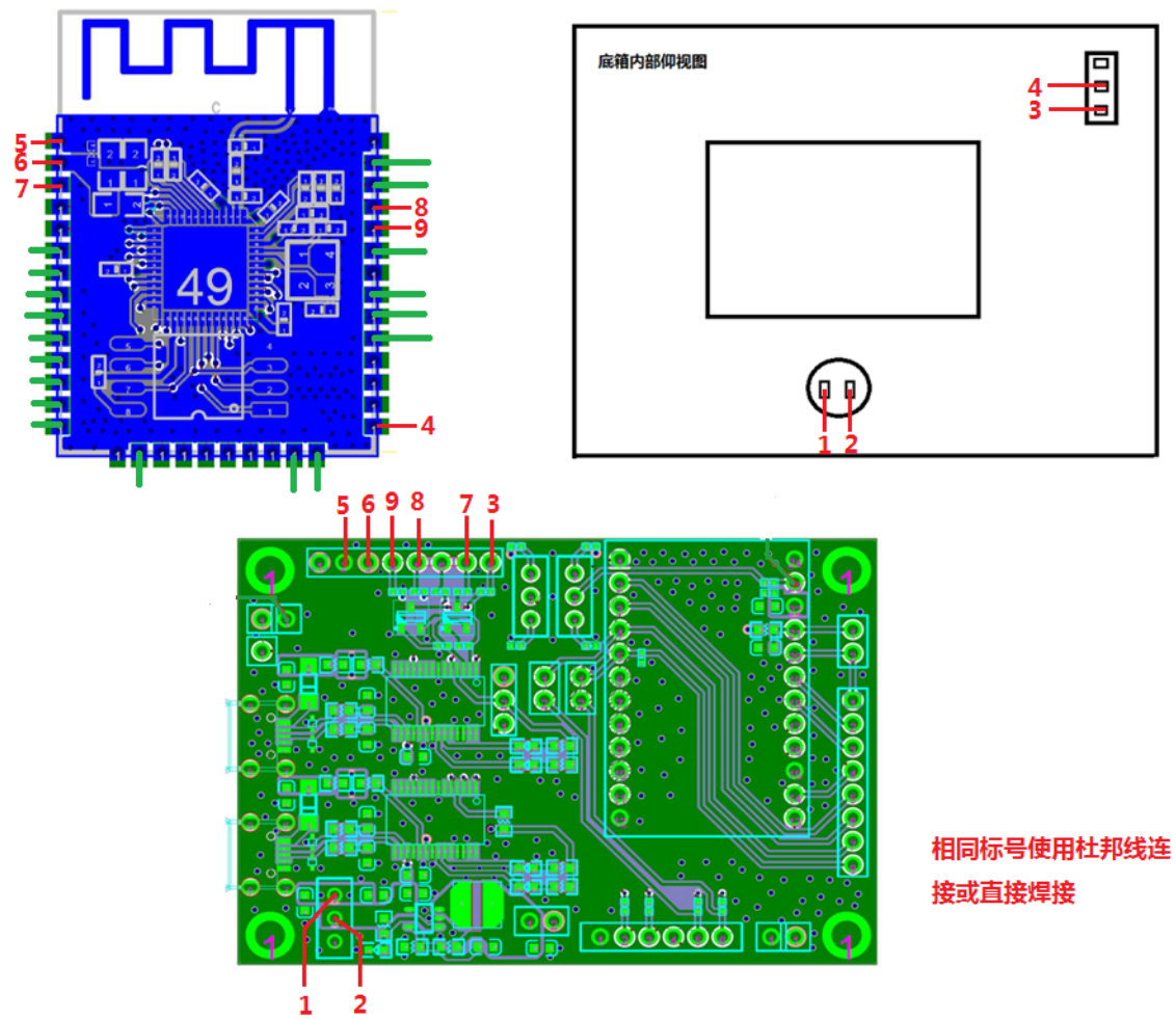
图 71: ESP-WROOM-32 模组台接线示意图
