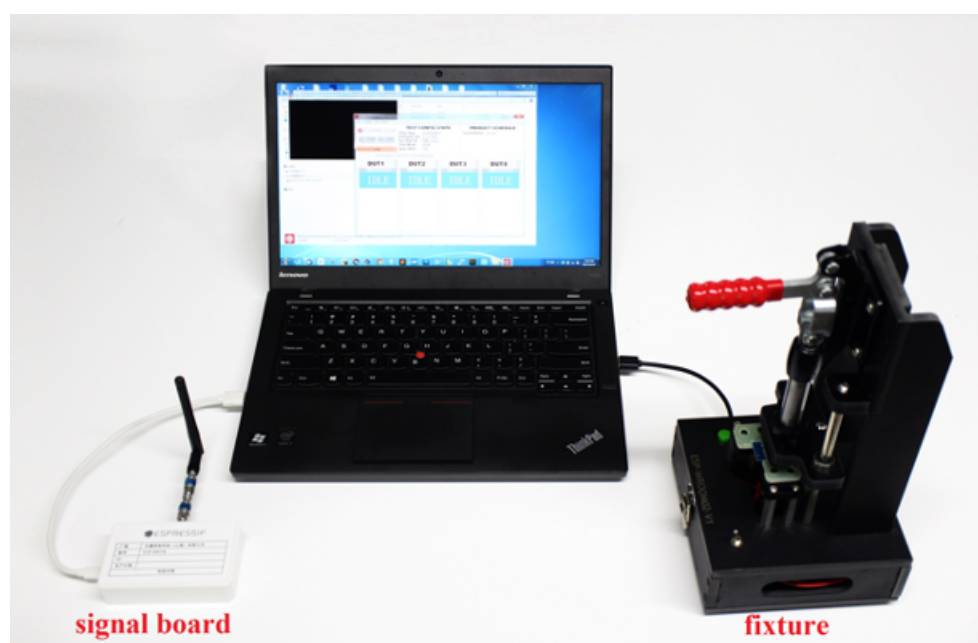
图 43: 信号板方案的实物连接
