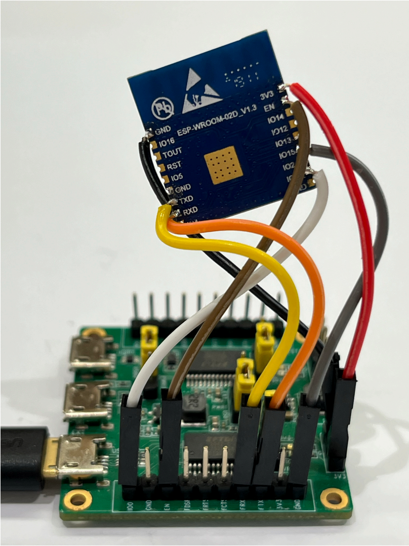
图 47: ESP32-WROOM-32D 模组接线图
