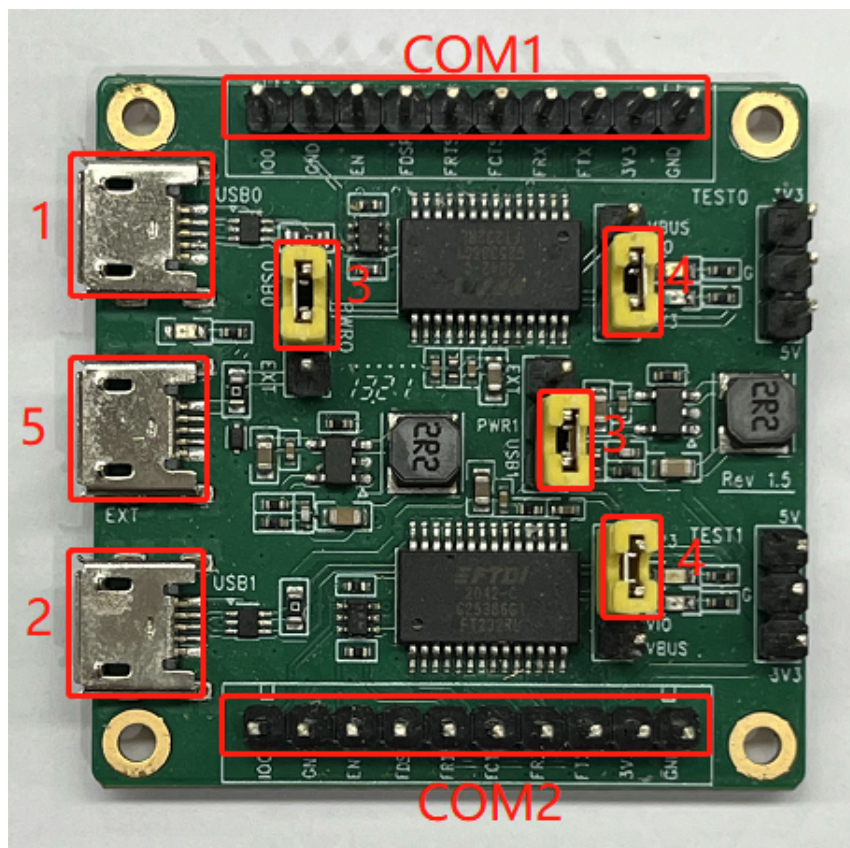
图 44: 串口底板示意图
