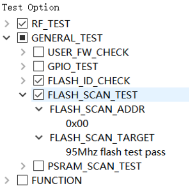
图 54: Flash 功能测试
