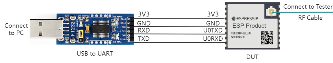
图 29: UART 连接说明
