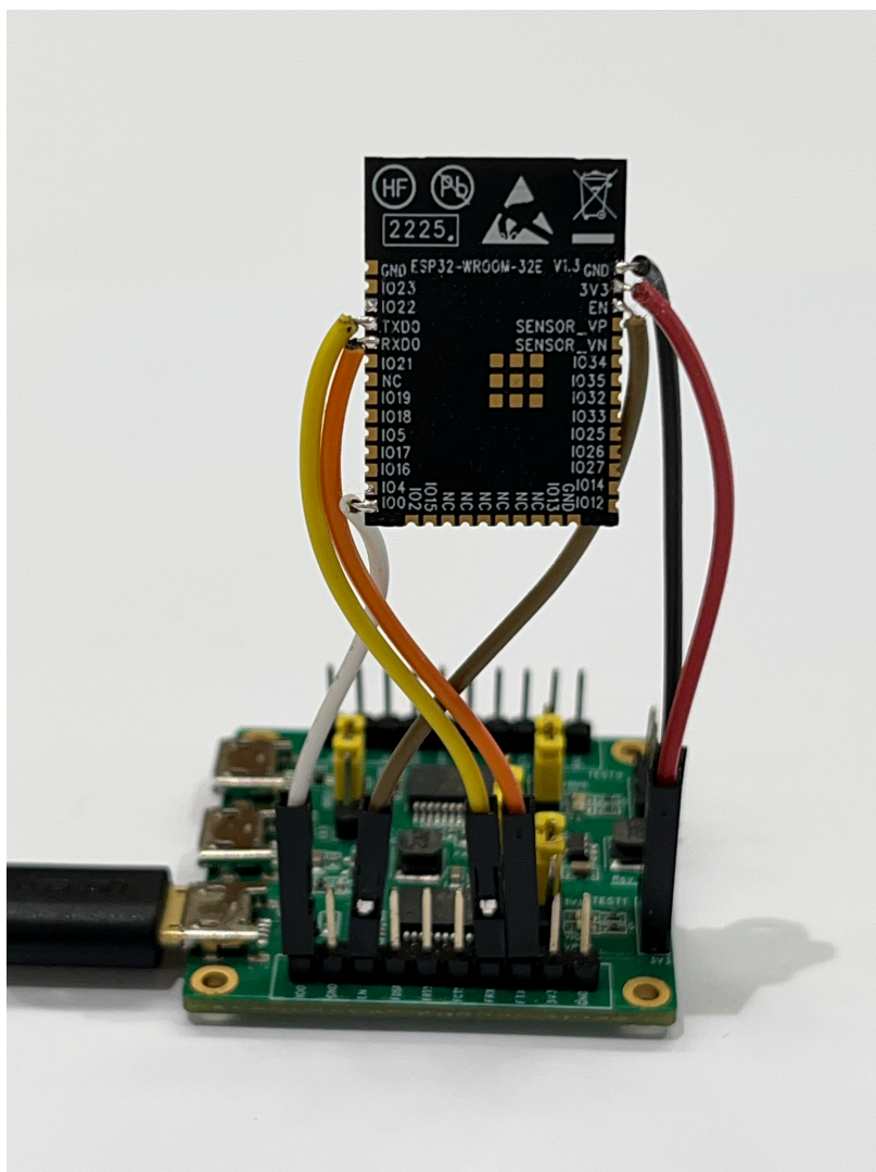
图 75: ESP32-WROOM-32E 模组接线图
