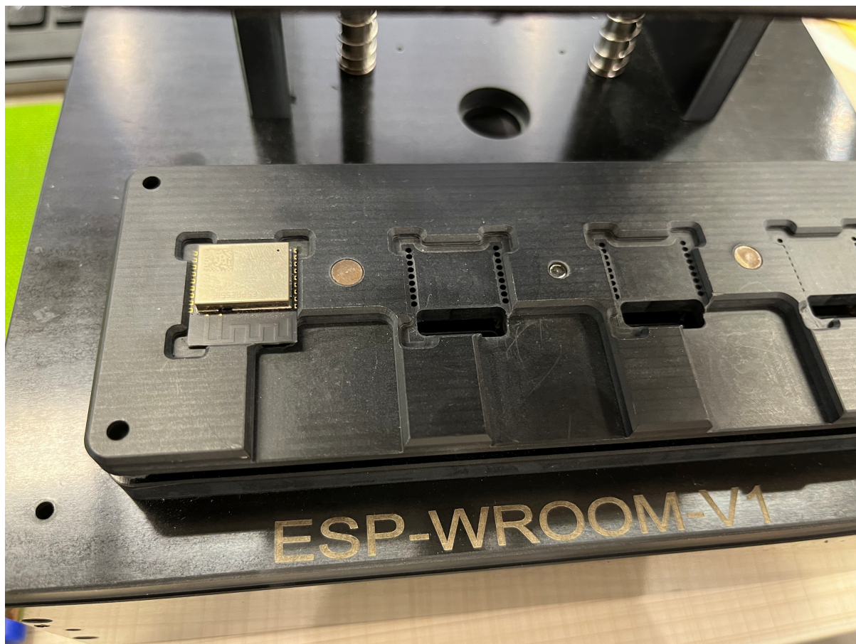
图 88: ESP-WROOM 治具模组台
