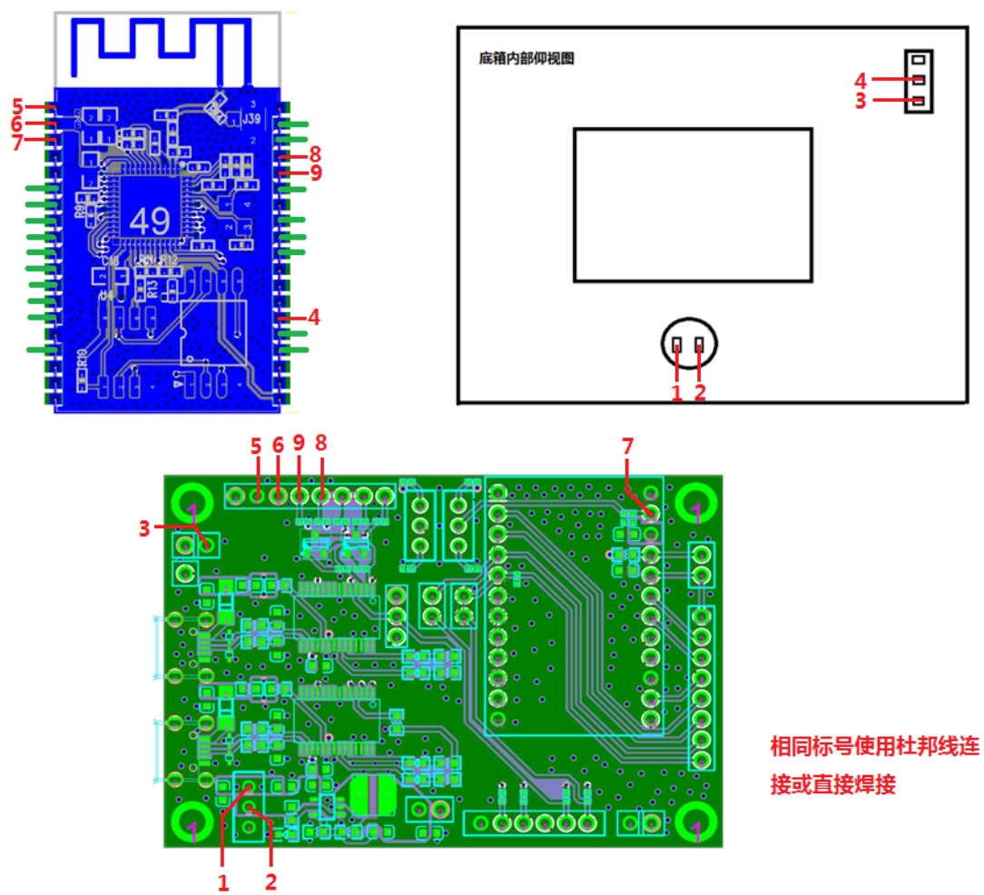
图 65: ESP32-WROOM-32 模组台接线示意图
