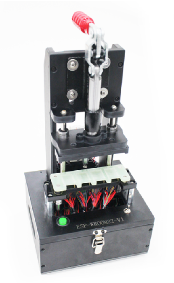
图 41: 治具整体外观
