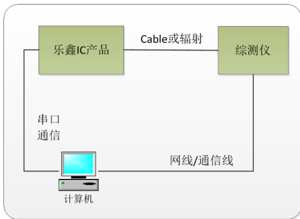
图 37: 仪器方案框架
