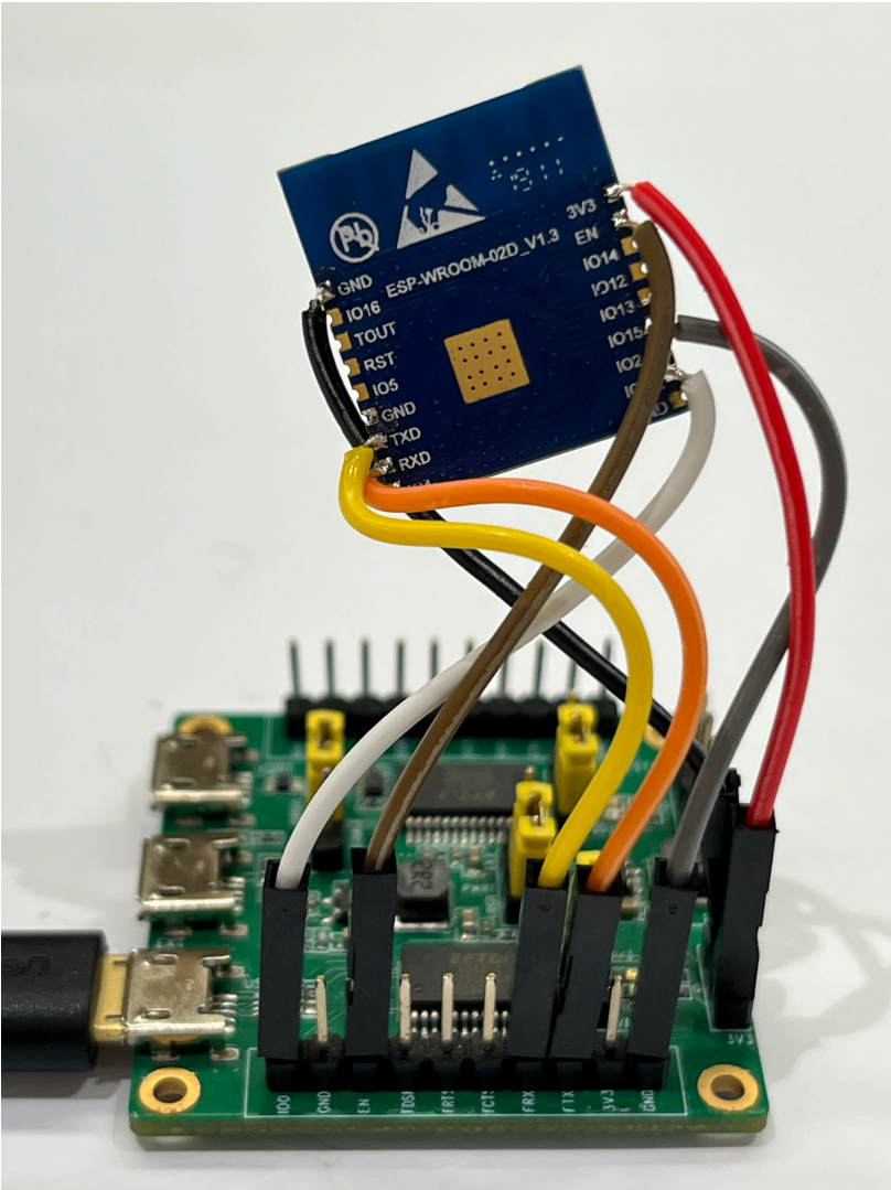
图 43: ESP32-WROOM-32D 模组接线图
