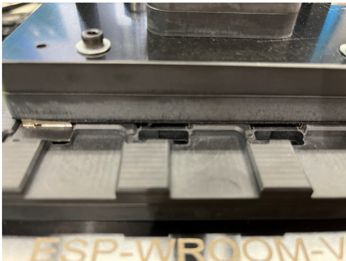
图 61: 活动台与模组台之间的距离示意
