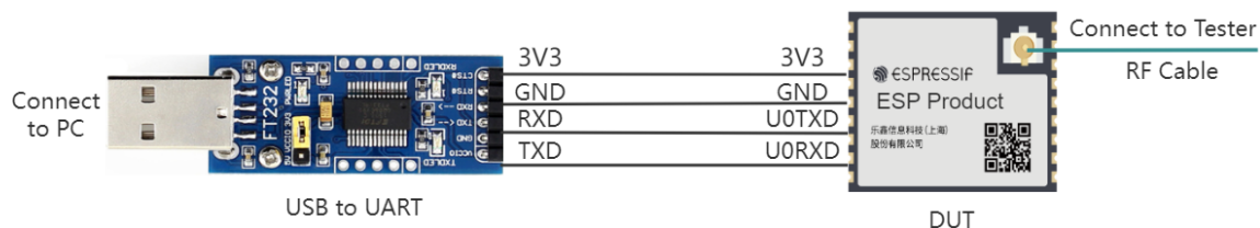
图 25: UART 连接说明
