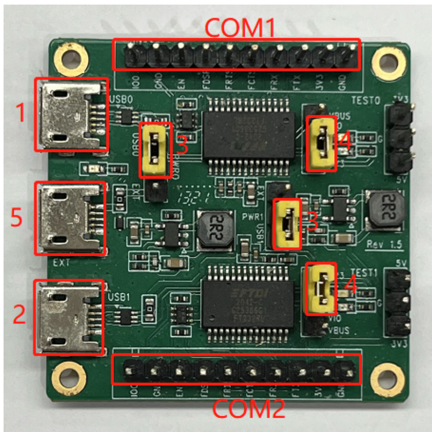
图 40: 串口底板示意图
