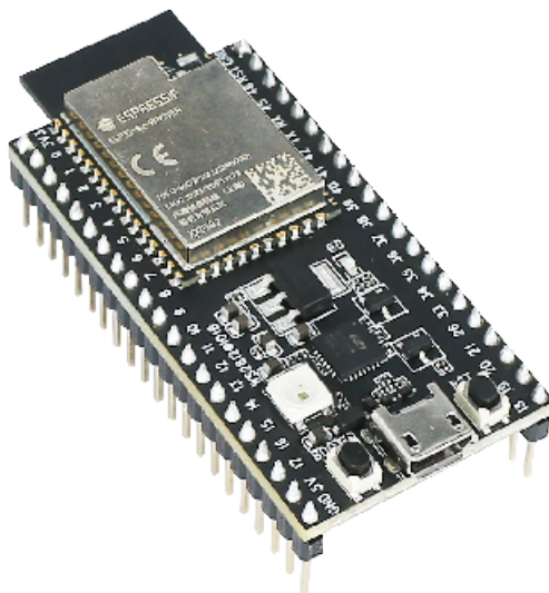
Fig. 51: ESP32-S2-Saola-1
