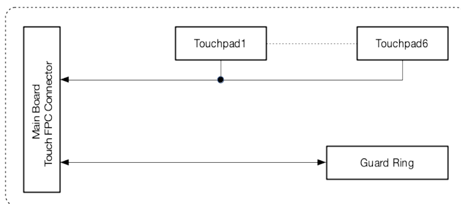
Fig. 37: ESP-LyraP-TouchA-v1.1 block diagram
