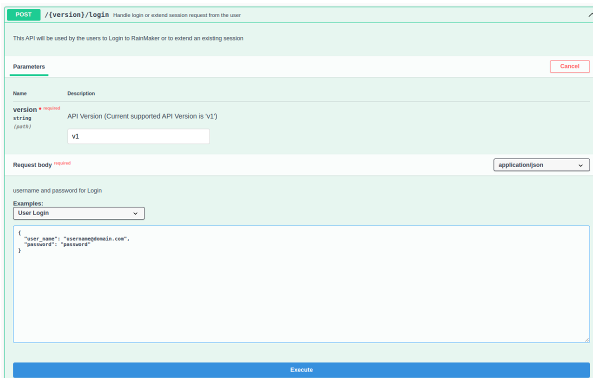
图 6: REST API 登陆
