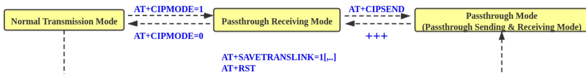
图 1: Transmission Mode Shift Diagram
