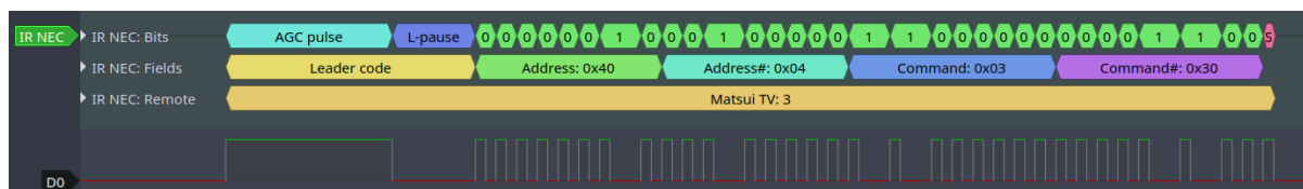
图 20: 红外 NEC 帧
