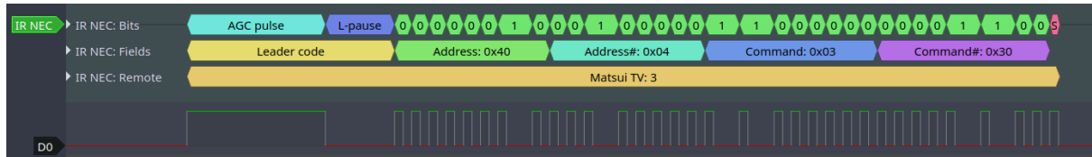
图 18: 红外 NEC 帧
