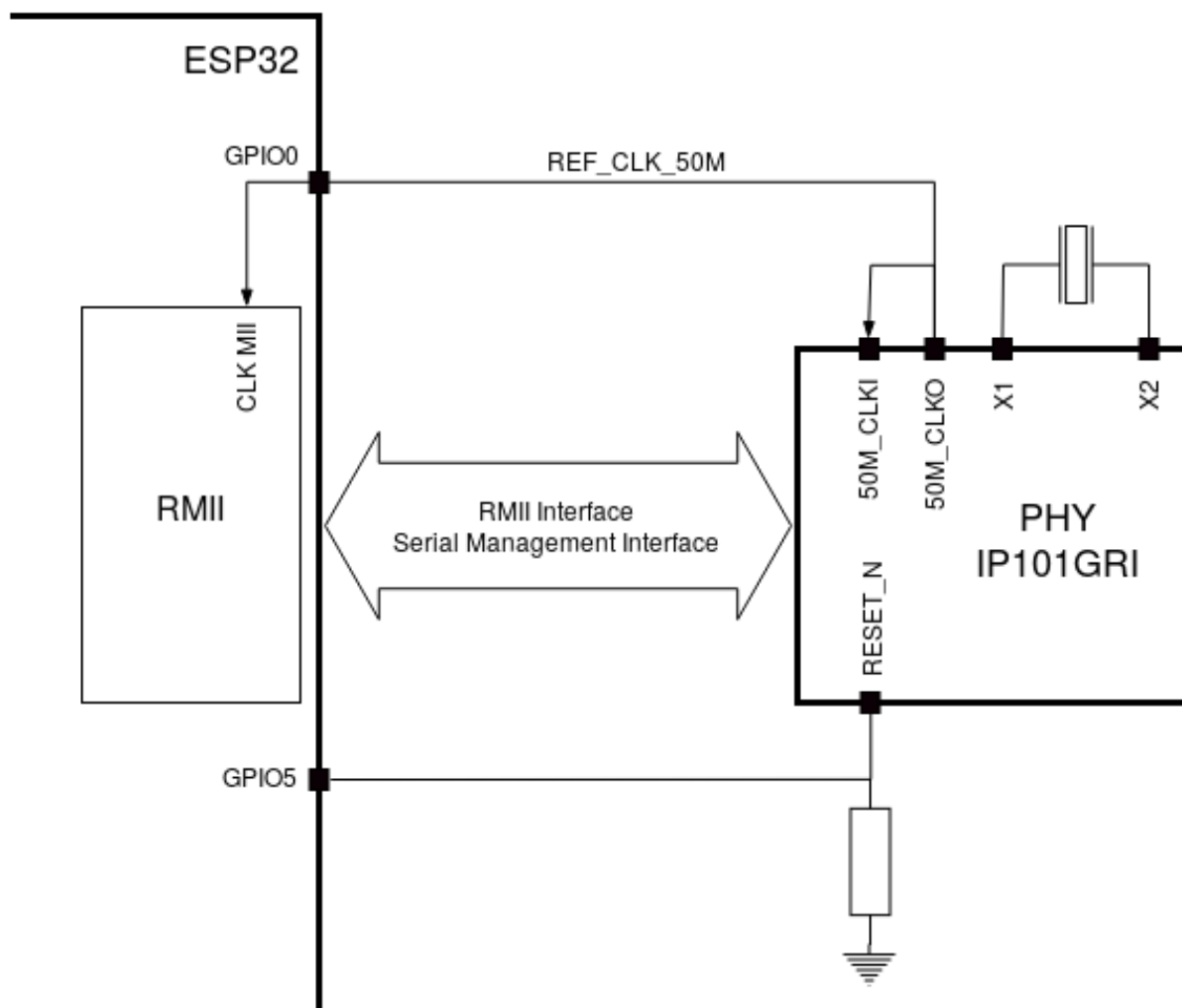
图 26: PHY 侧提供 RMIIClock 时钟
