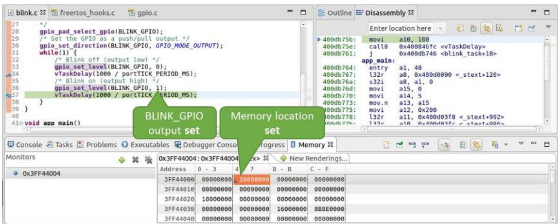
图 53: 观察内存地址 0x3FF44004 处的某个比特被置高
