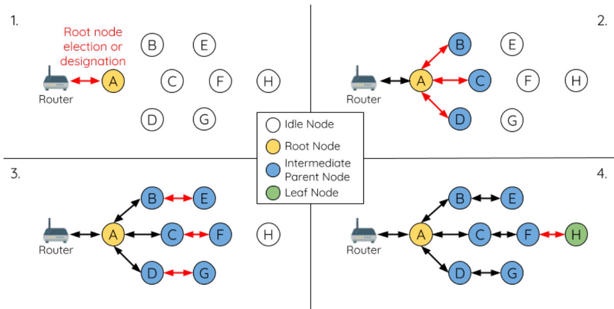
图 30: ESP-WIFI-MESH 网络构建过程
