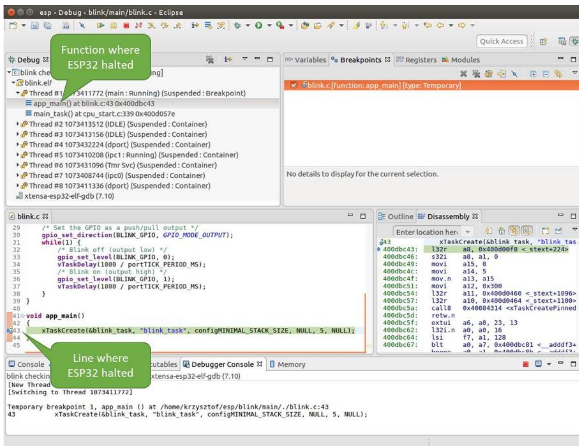
图 46: 调试时目标停止
