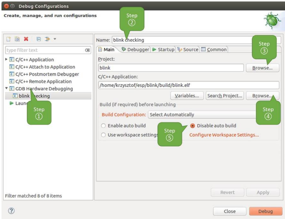
图 41: GDB 硬件调试的配置 - Main 选项卡
