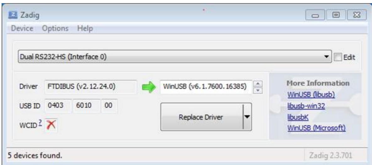
图 40: 在 Zadig 工具中配置 JTAG USB 驱动
