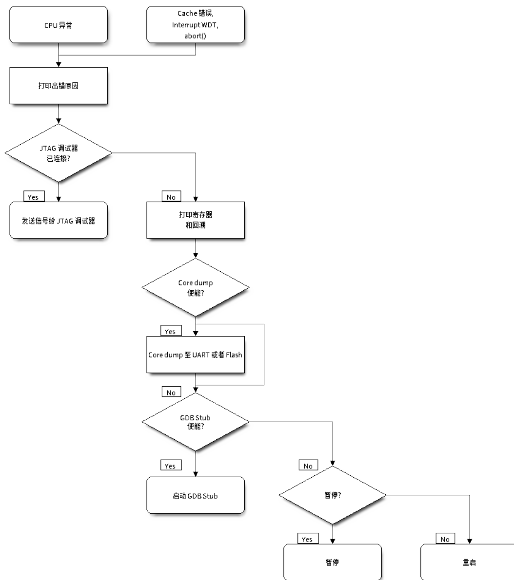
图 38: 紧急处理程序流程图 (点击放大)
