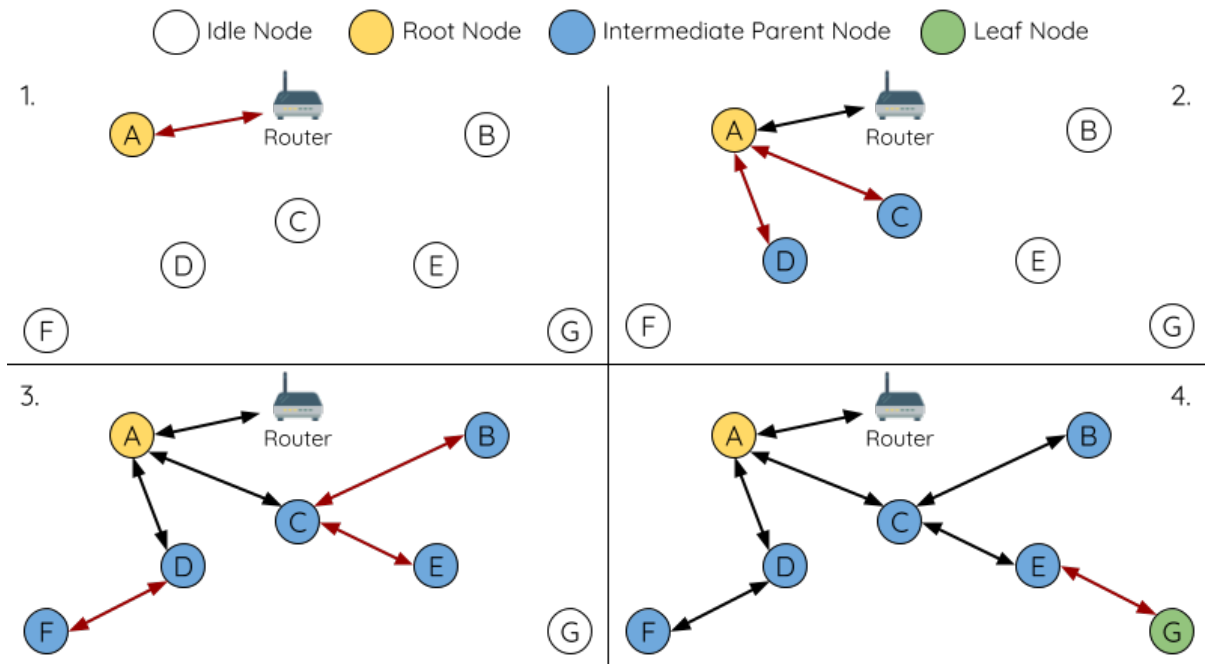
图 32: 根节点指定示例 (根节点 = A, 最大层级 = 4)
