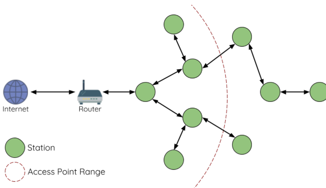
图 24: ESP-WIFI-MESH 网络架构示意图
