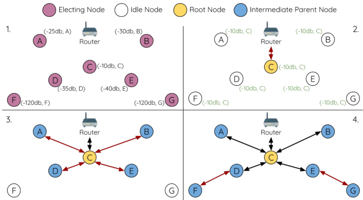
图 31: 根节点选举示例
