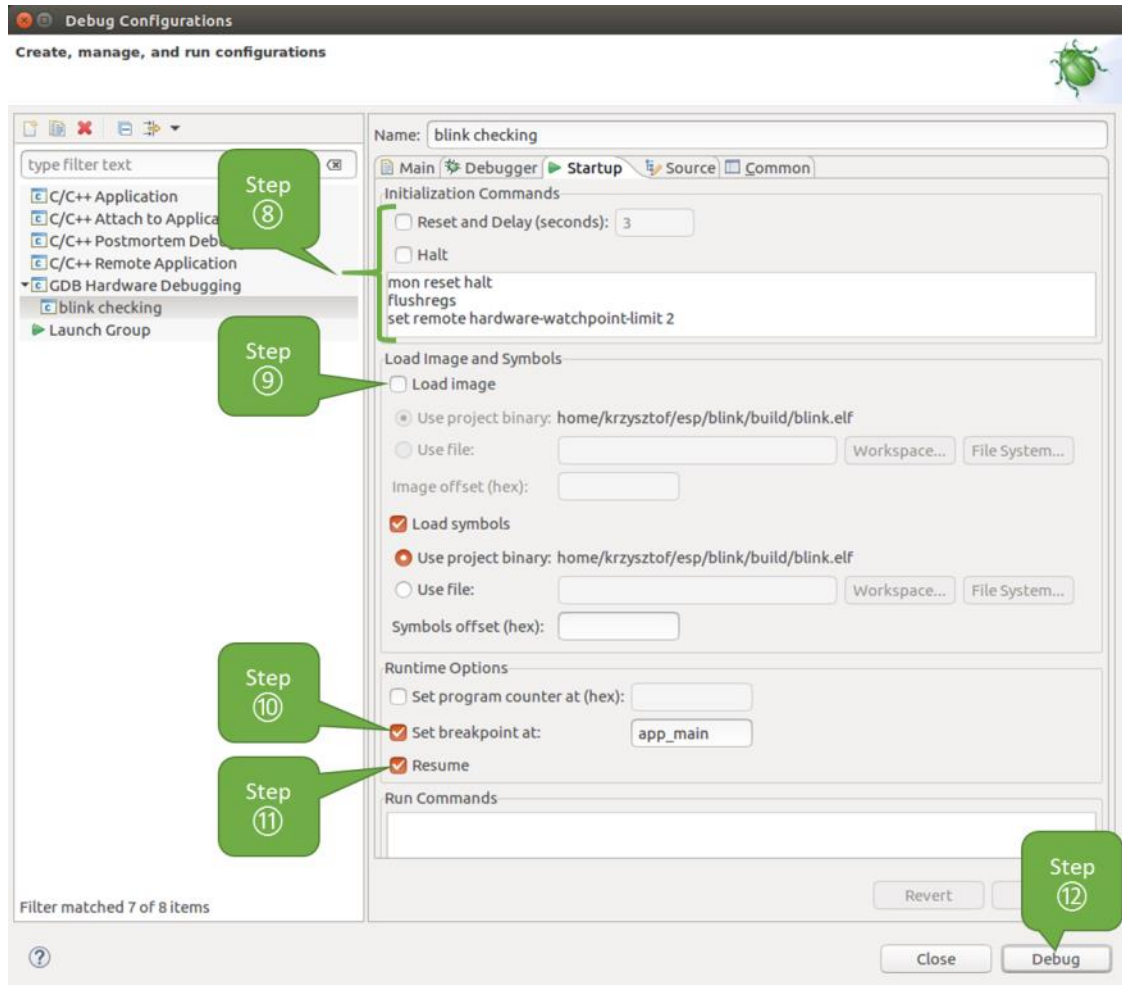
图 43: GDB 硬件调试的配置 - Startup 选项卡
