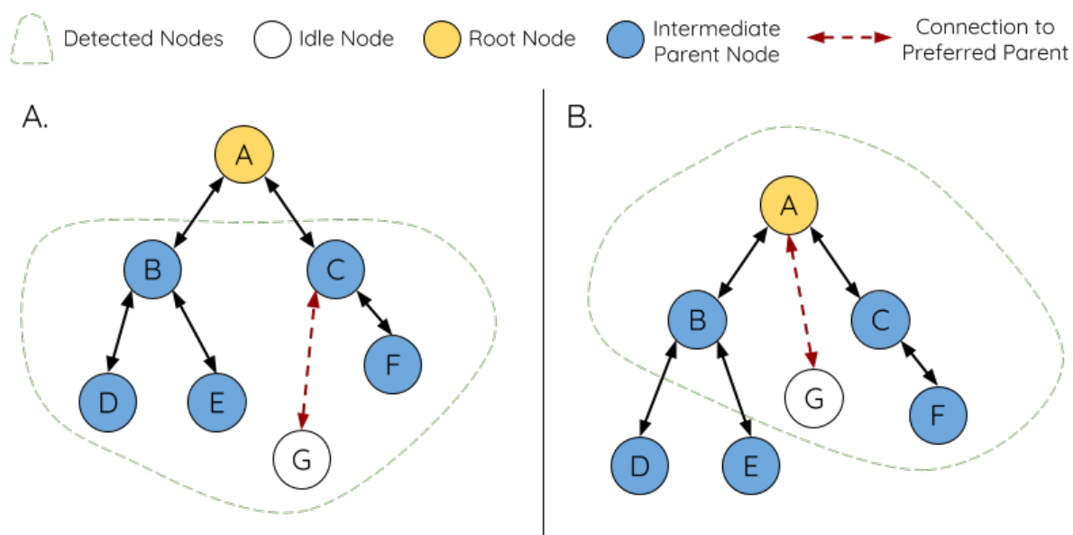
图 28: 首选父节点选择
