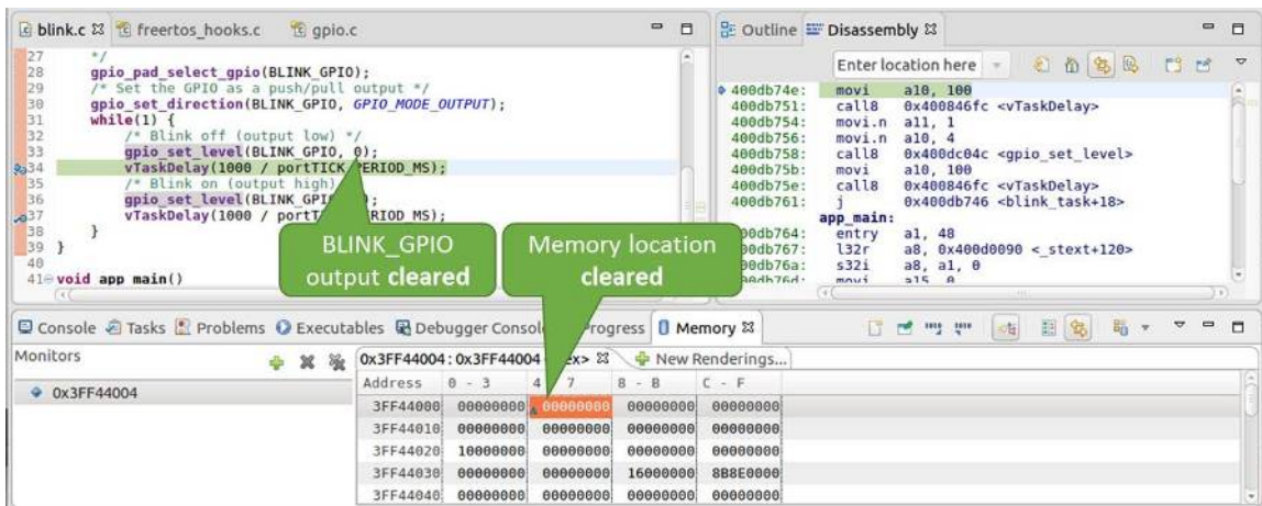
图 54: 观察内存地址 0x3FF44004 处的某个比特被置低
