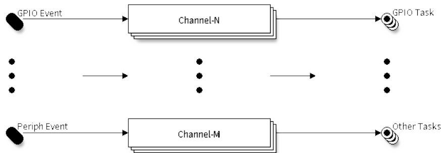
图 3: ETM 通道概述
