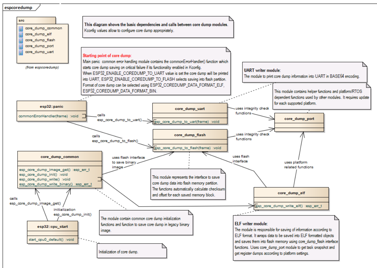
图 6: 核心转储实现
