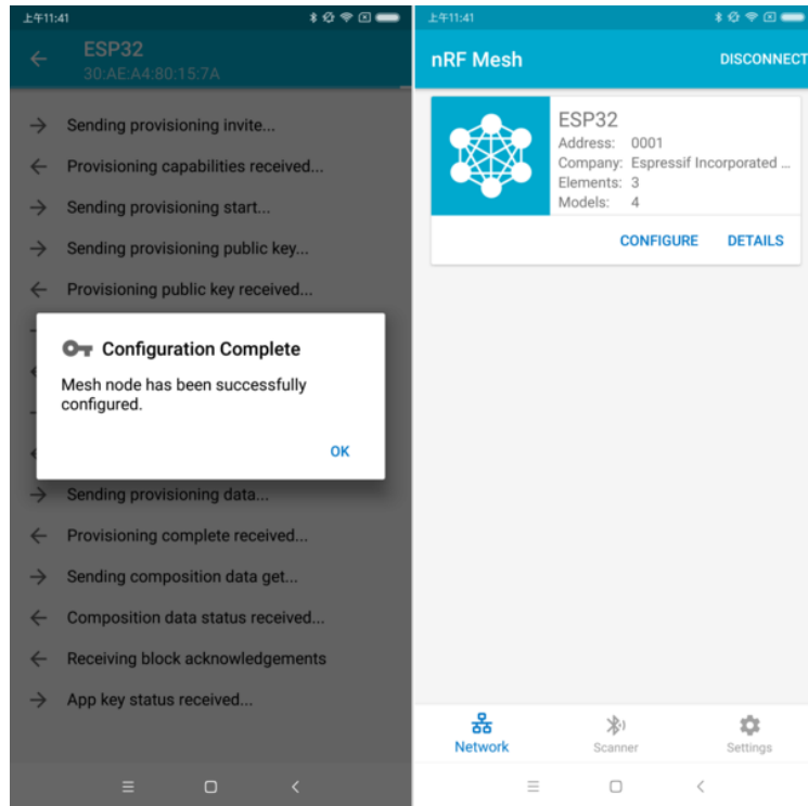
图 13: nRF Mesh - 配置完成
