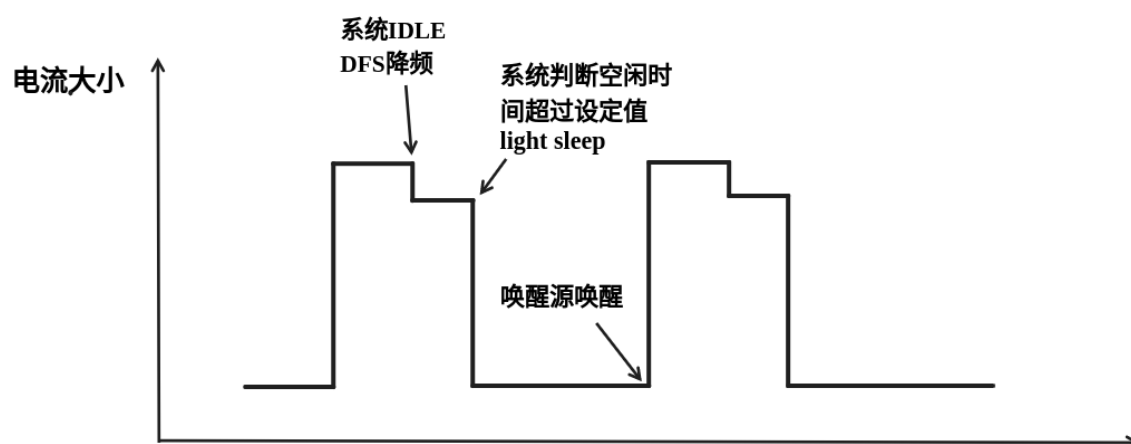
图 43: Auto Light-sleep 模式模式理想电流图
