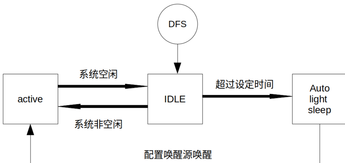
图 42: Auto Light-sleep 模式工作流程图
