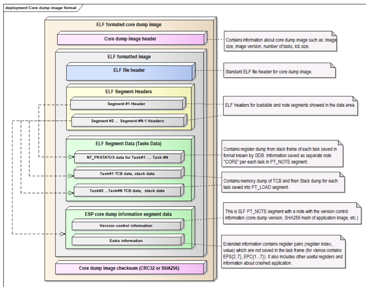
图 4: 核心转储 ELF 镜像文件格式
