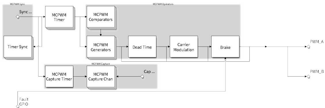
图 15: MCPWM 概述
